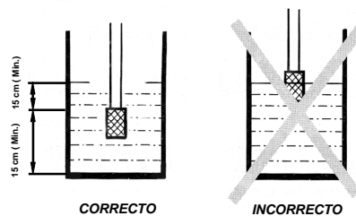
Figura 2 : Posición de la válvula de pie
