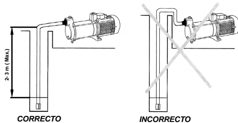
Figura 1 : Aspiración
