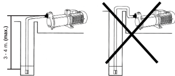
Figura 1: Aspiración
