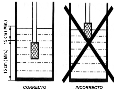
Figura 2 : Posición de la válvula de pie
