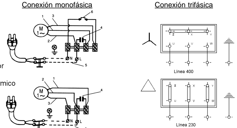
Figura 3 : Conexiones eléctricas
