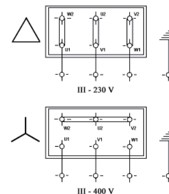
Figura 3: Conexión eléctrica
