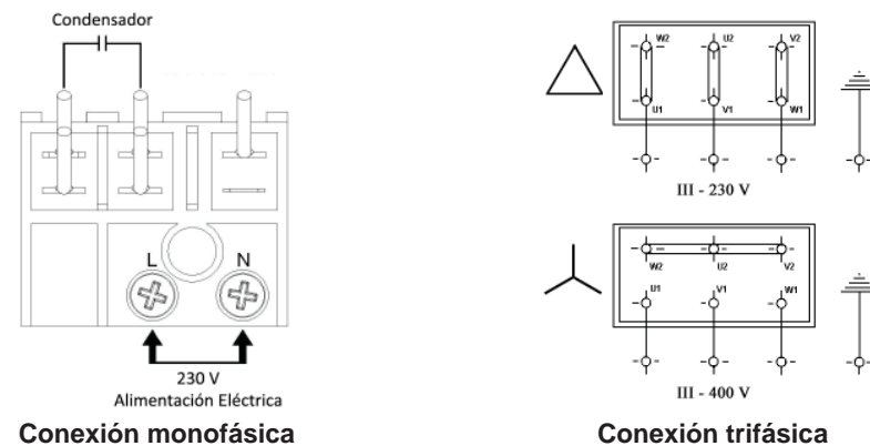
Figura 3: Conexiones eléctricas
