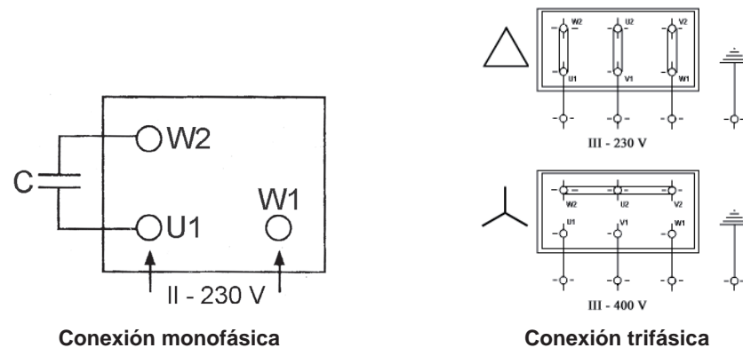
Figura 3: Conexiones eléctricas
