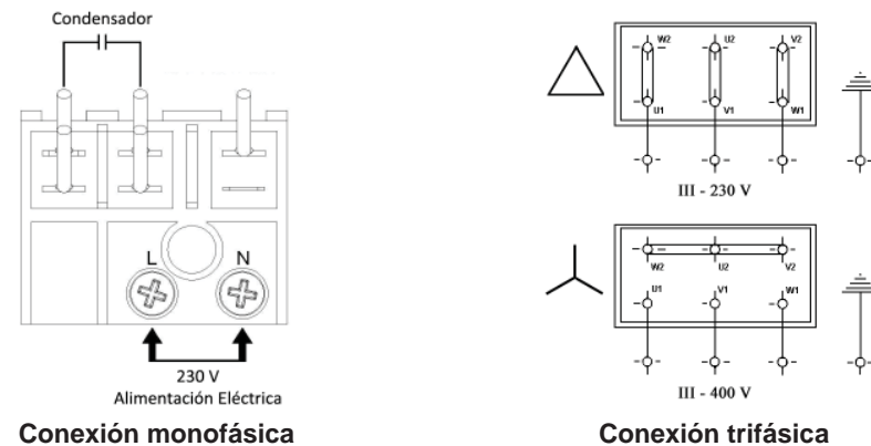
Figura 3: Conexiones eléctricas
