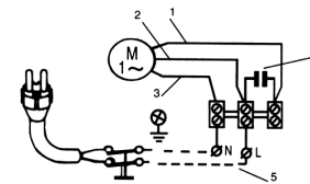
Figura 3 : Conexiones eléctricas
