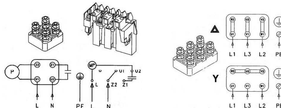
Conexión monofásica
