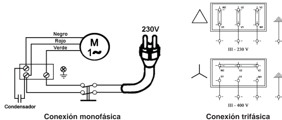
Figura 3: Conexiones eléctricas
