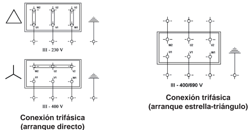
Figura 3: Conexiones eléctricas
