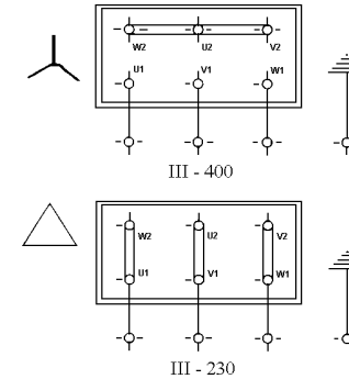
Figura 3 : Conexión trifásica
