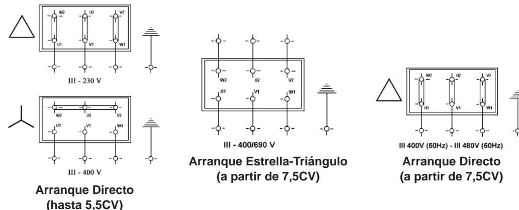
Figura 3: Conexiones eléctricas
