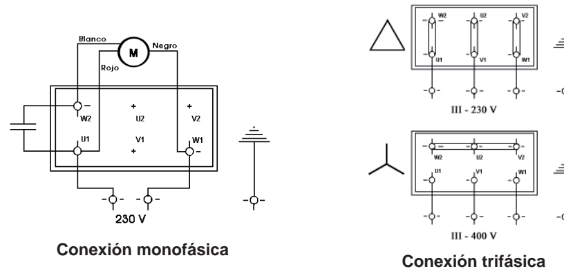
Figura 3: Conexiones eléctricas
