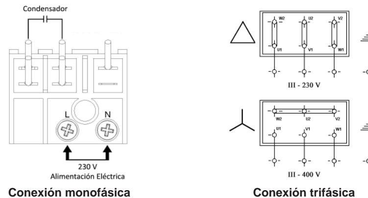
Figura 3: Conexiones eléctricas
