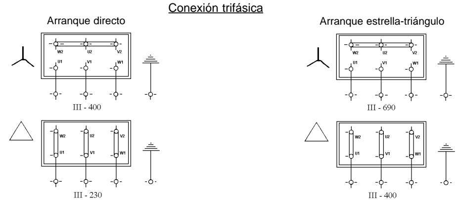
Figura 3 : Conexiones eléctricas
