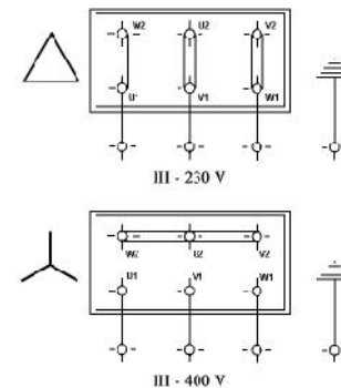
Figura 3: Conexiones eléctricas
