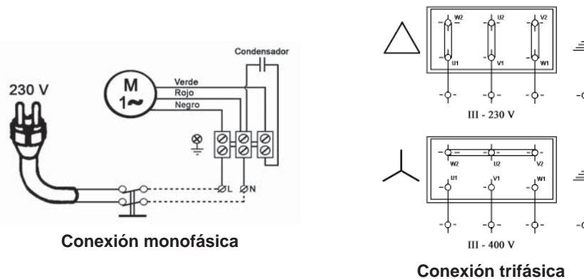
Figura 3: Conexiones eléctricas
