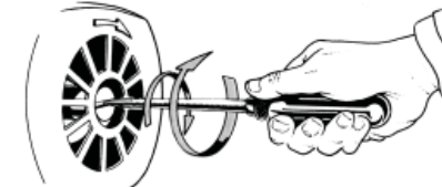
Figura 4: Desbloquear eje
