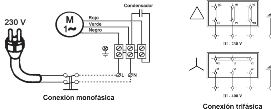
Figura 3: Conexiones eléctricas
