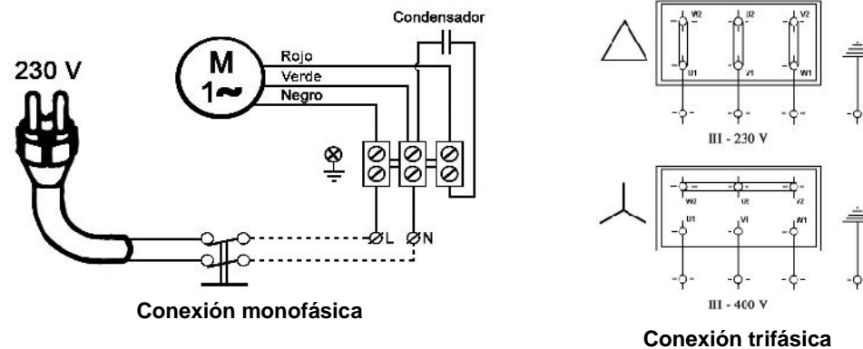
Figura 3: Conexiones eléctricas
