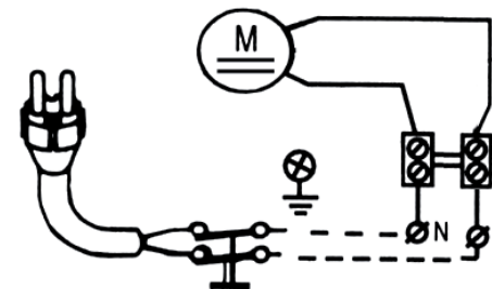
Figura 3: Conexión eléctrica
