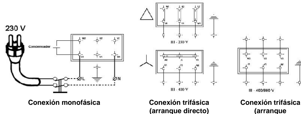
Figura 3: Conexiones eléctricas
