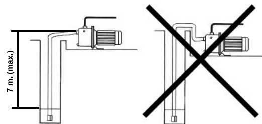
Figura 1: Aspiración
