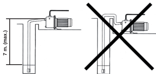
Figura 1: Aspiración
