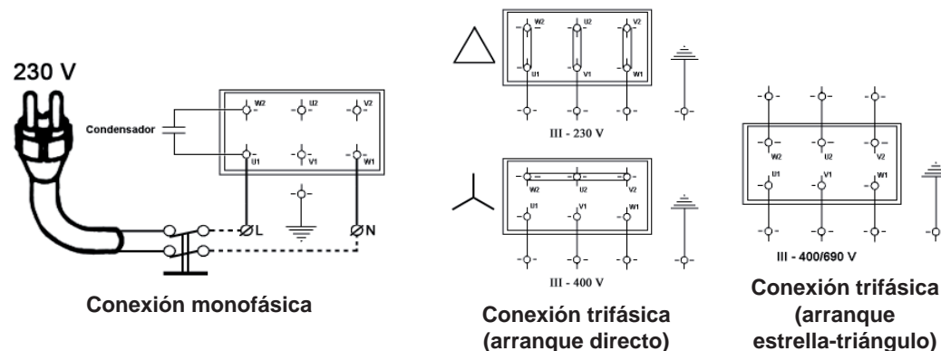
Figura 3: Conexiones eléctricas
