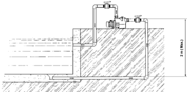
Figura 1 : Instalación
