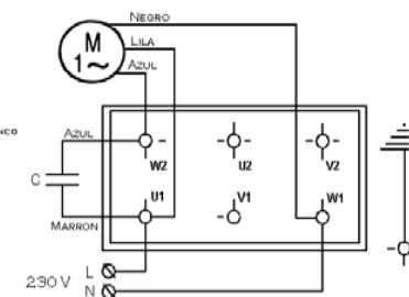
Figura 3 : Conexiones eléctricas
