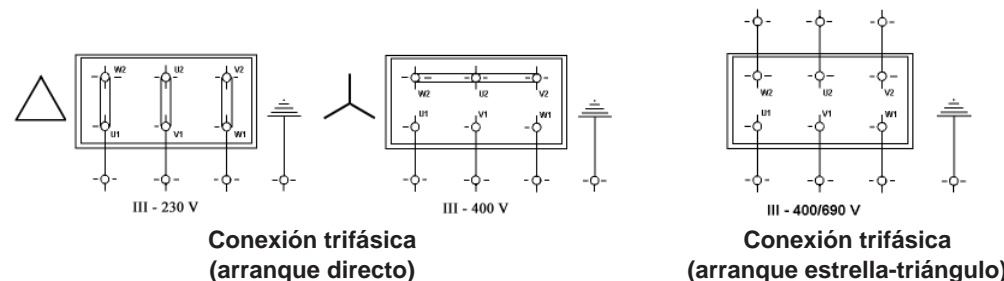
Figura 2: Conexiones eléctricas
