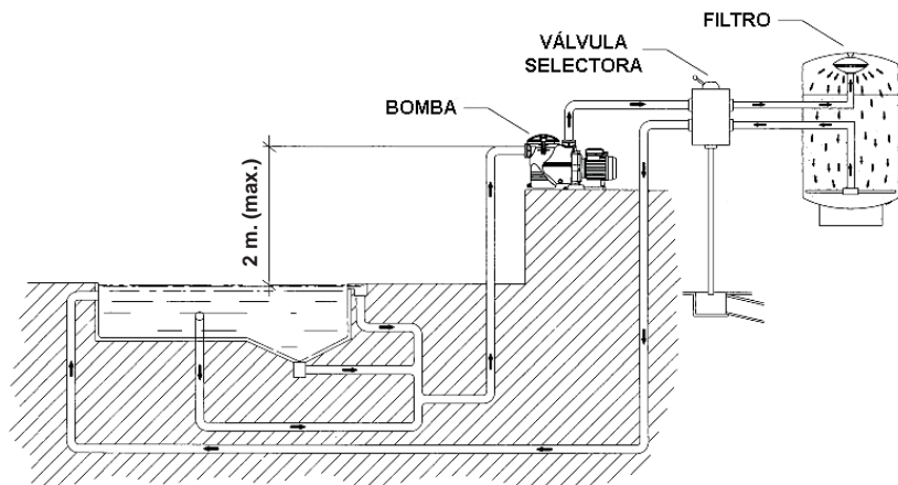
Figura 1: Instalación
