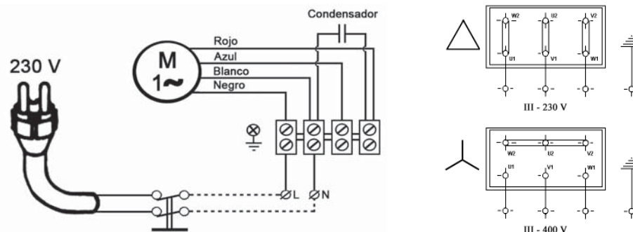
Conexión monofásica
