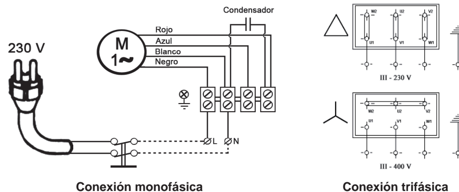
Figura 3: Conexiones eléctricas
