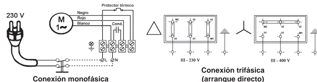
Figura 2: Conexiones eléctricas
