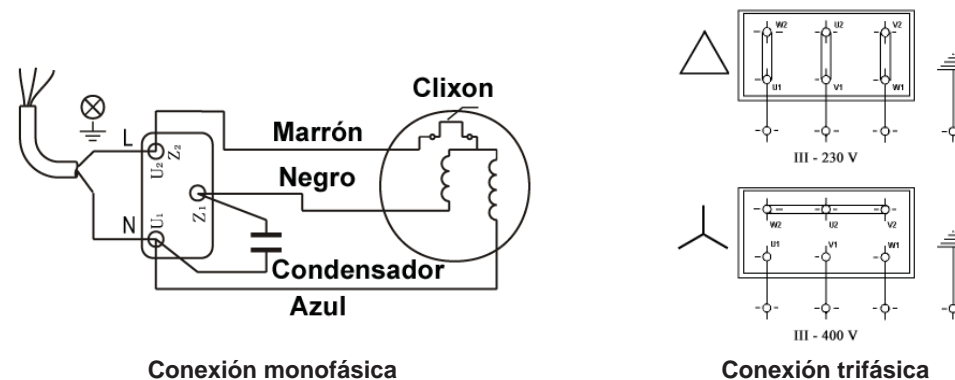
Figura 3: Conexiones eléctricas
