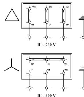
Figura 3: Conexión trifásica
