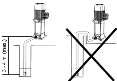
Figura 1: Aspiración
