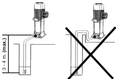
Figura 1: Aspiración
