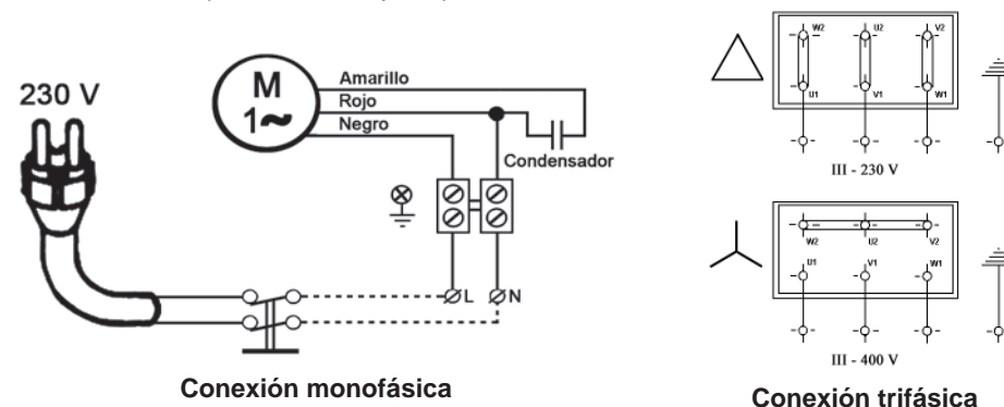
Figura 3: Conexiones eléctricas
