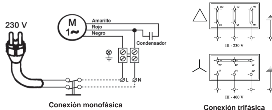
Figura 3: Conexiones eléctricas
