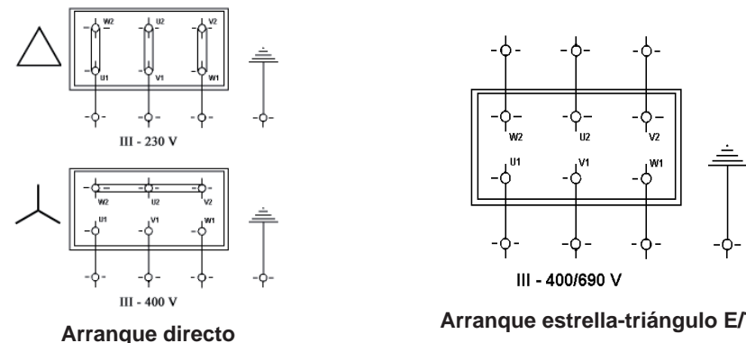
Figura 3: Conexión trifásica
