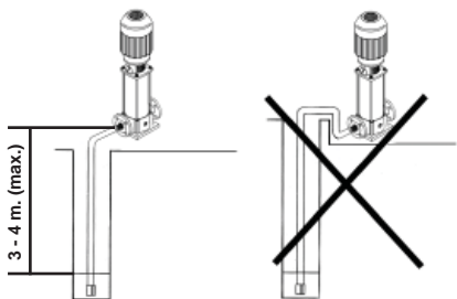
Figura 1: Aspiración
