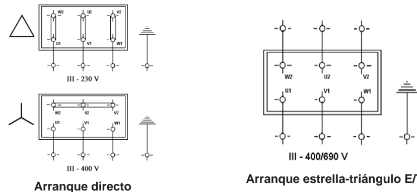
Figura 3: Conexión trifásica
