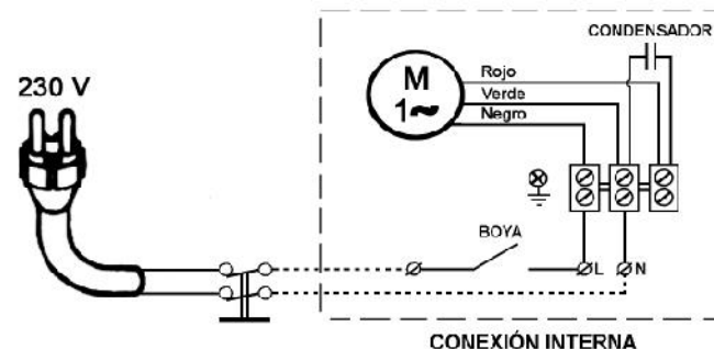
Figura 3: Conexión monofásica
