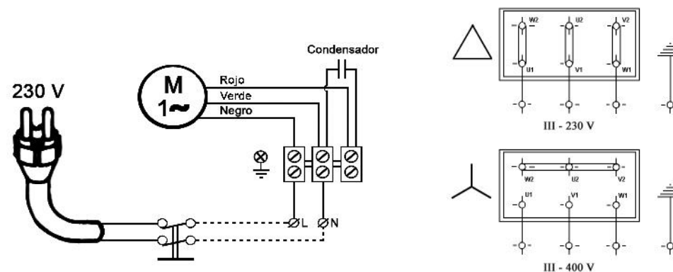
Conexión monofásica
