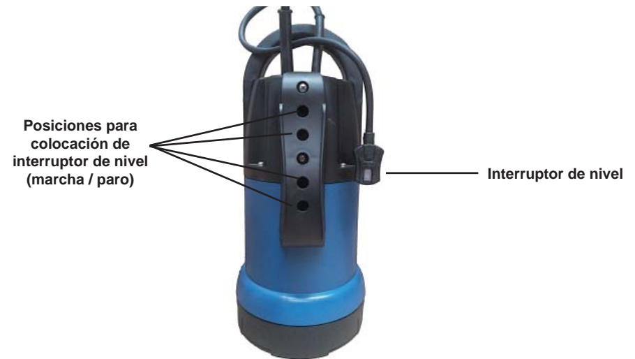
Figura 3 : Interruptor de nivel
