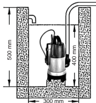
Figura 2 : Dimensiones mínimas aconsejadas
