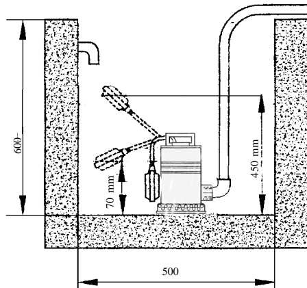
Figura 2 : Dimensiones mínimas útiles aconsejadas
