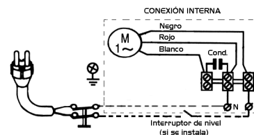
Figura 3 : Conexión MOPA-40 M
