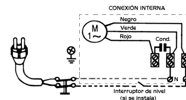
Figura 4 : Conexión MOPA-50 M
