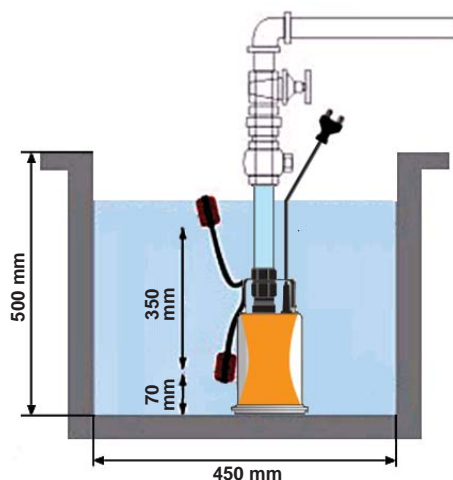
Dimensiones mínimas
