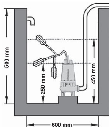
Dimensiones mínimas
