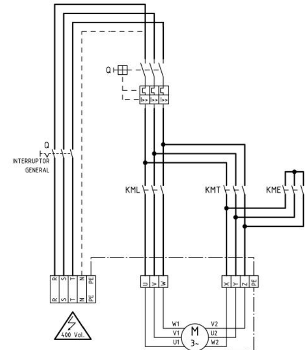
FIG.7 - Conexión trifásica (arranque estrella - triángulo)
