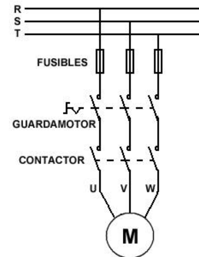
FIG.6 - Conexión trifásica (arranque directo)
