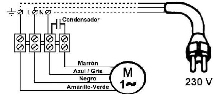
FIG. 5 - Conexión monofásica
