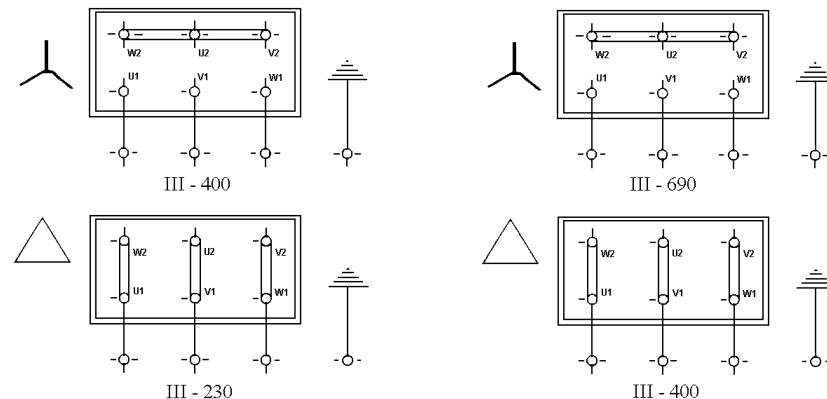
Figura 3 : Conexión trifásica
