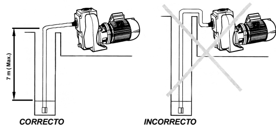
Figura 1 : Aspiración
