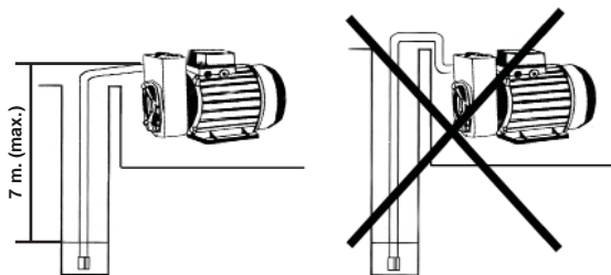
Figura 1: Aspiración
