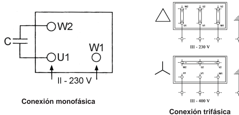
Figura 3: Conexiones eléctricas
